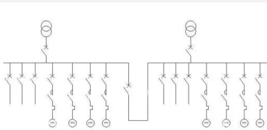
将若干个回路组合装配成低压开关柜
