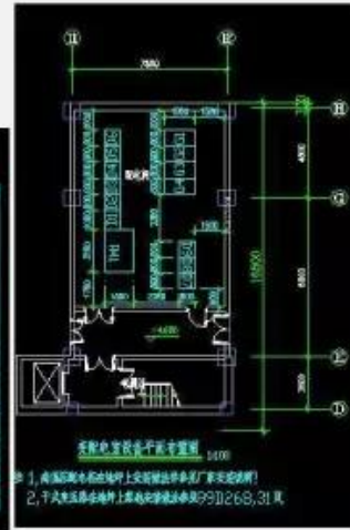
变配电室设备平面布置图
