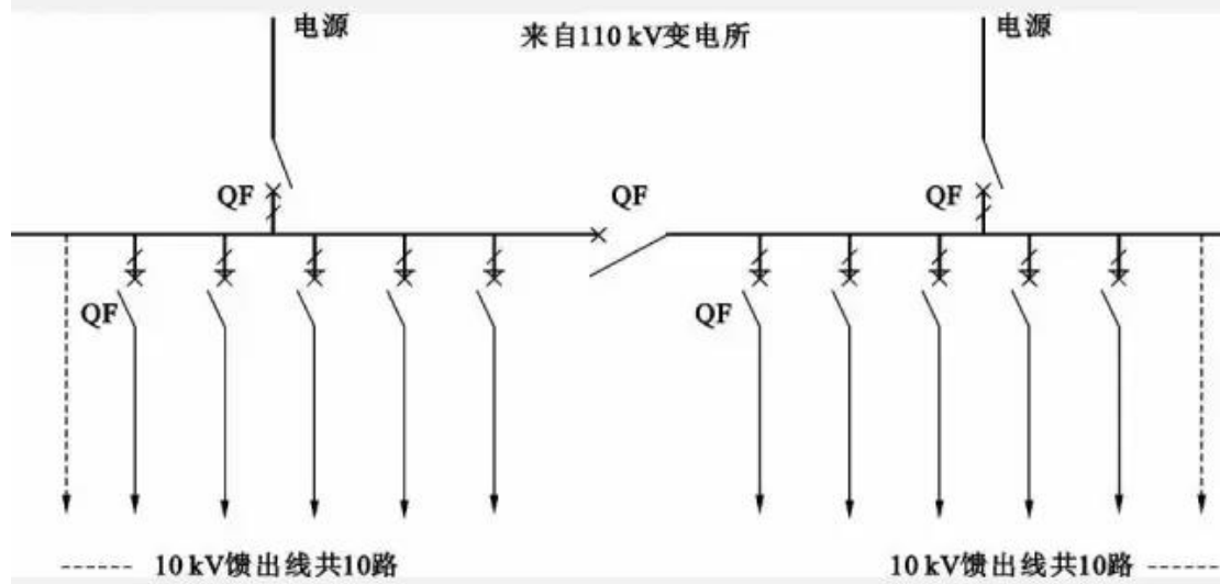
中压开闭所接线方式图
